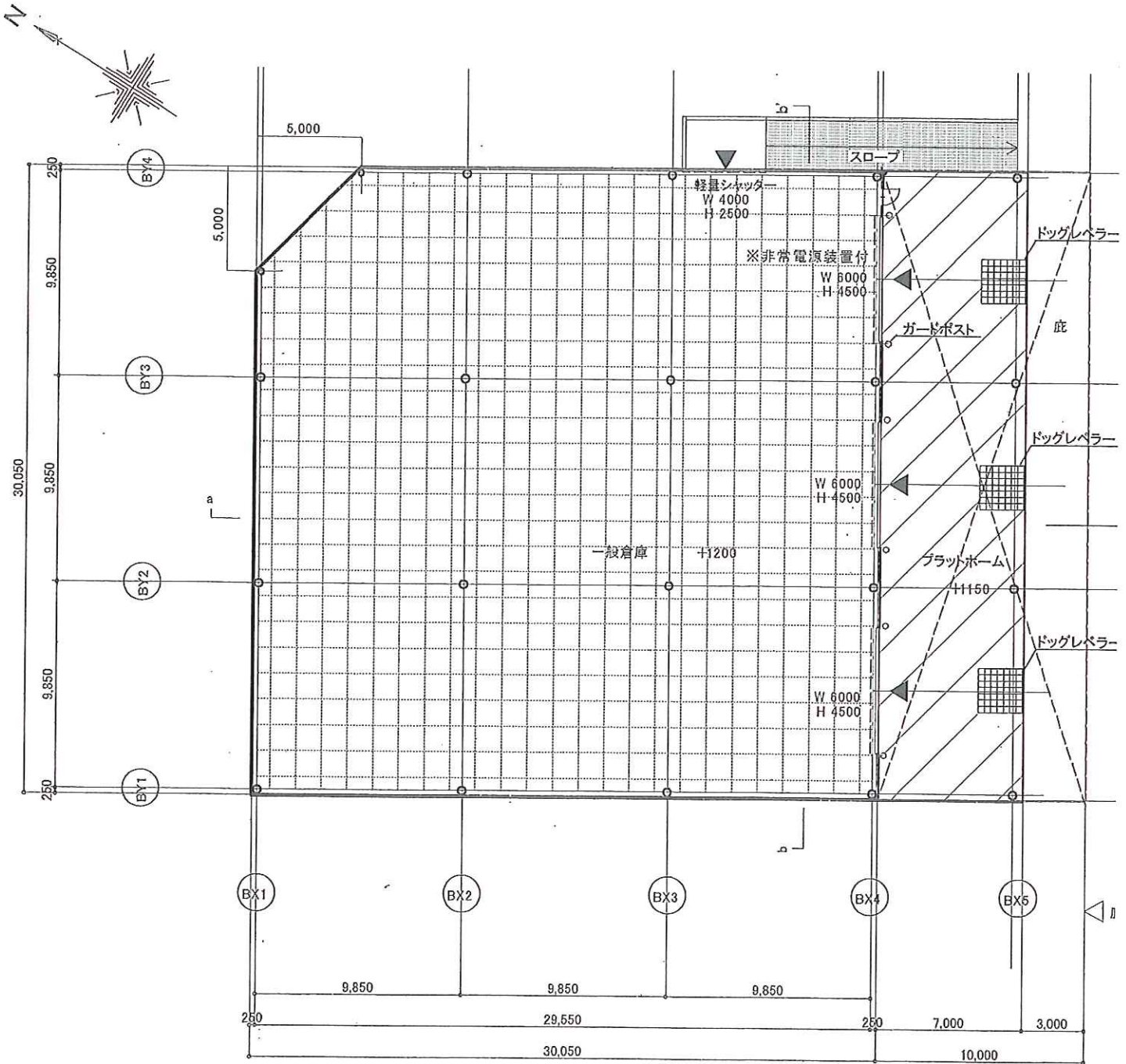
一般倉庫棟 平面図 1/200
