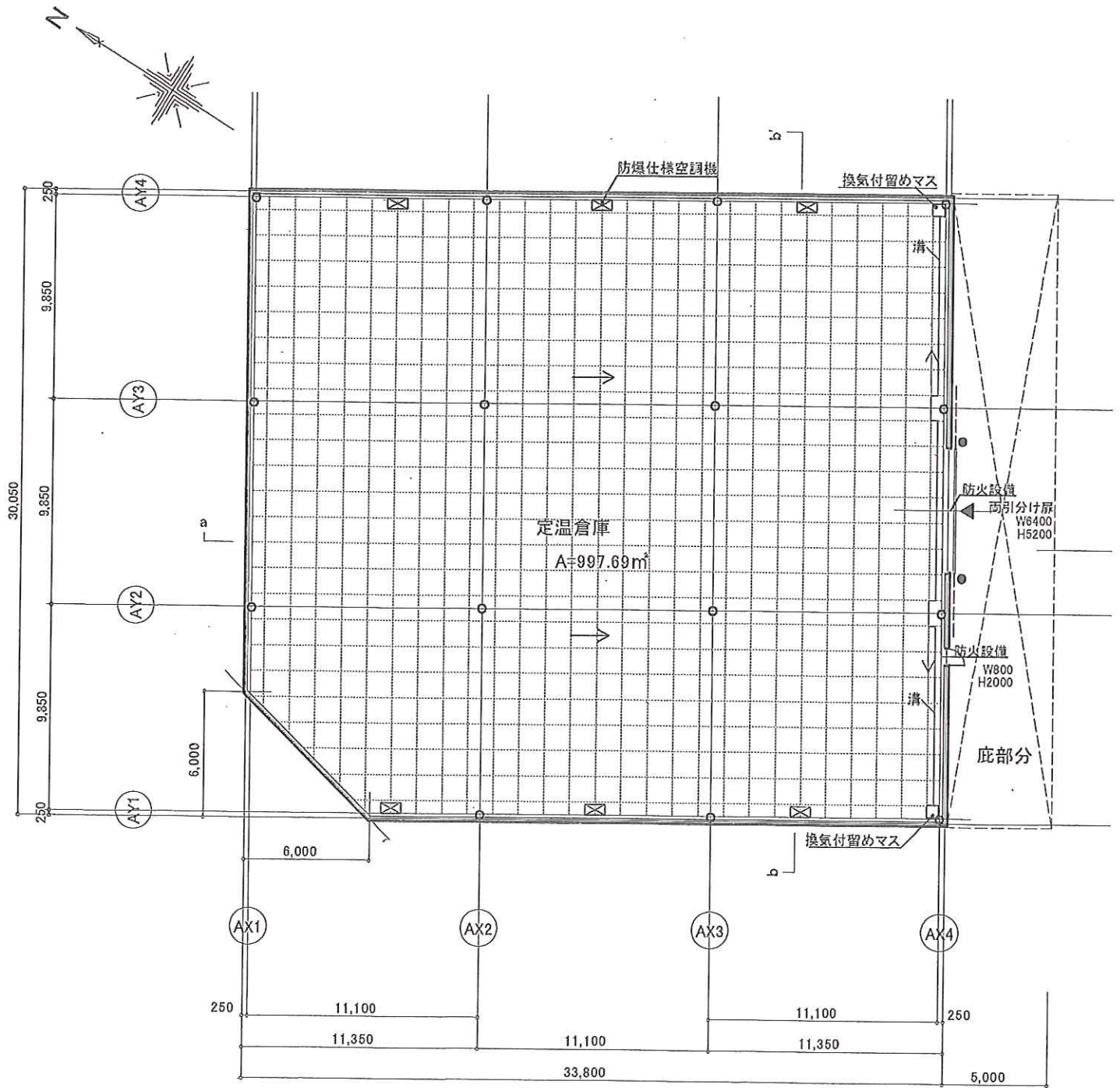
定温倉庫棟 平面図 1/200
